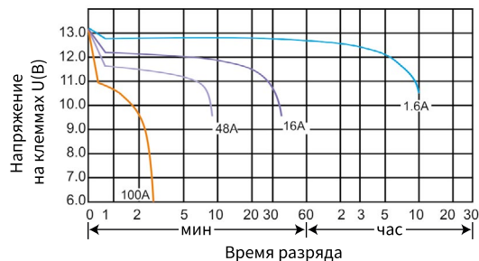
Разрядные характеристики
