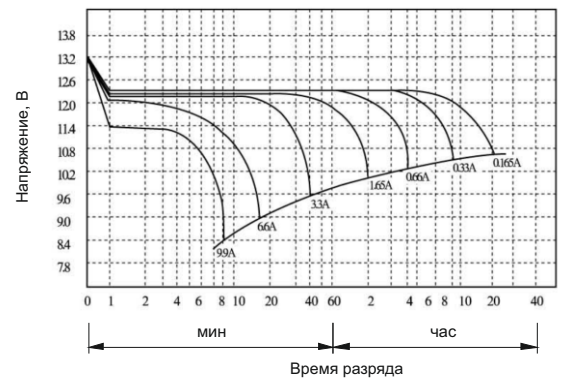
Разрядные характеристики
