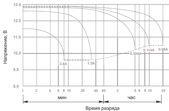
Разрядные характеристики
